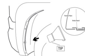
J-Clip
